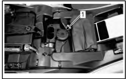
1. Компенсационный бачок заднего тормоза
