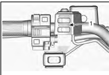
1. Светодиодный индикатор уровня обогрева
