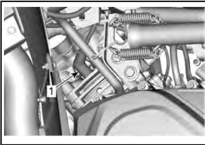
ПРАВАЯ СТОРОНА – ЗАДНИЙ ЦИЛИНДР 1. Свеча зажигания
