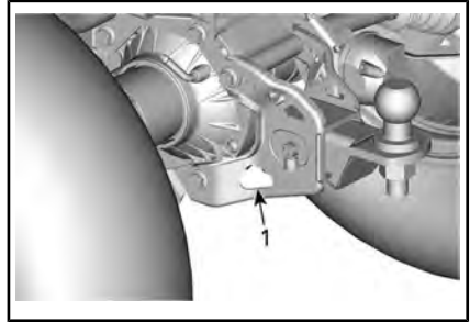
ТИПИЧНЫЙ ВАРИАНТ - РАСПОЛОЖЕНИЕ ЗАДНЕЙ ТОЧКИ КРЕПЛЕНИЯ
