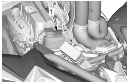
1. Расширительный бачок системы охлаждения
