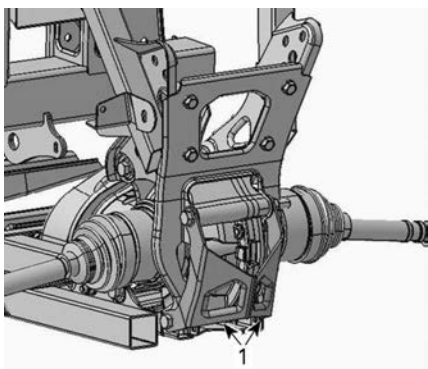
1. Буксировочные проушины
