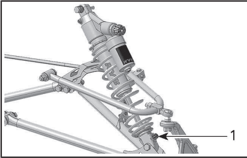
1. Рукоятка регулировки хода отбоя
