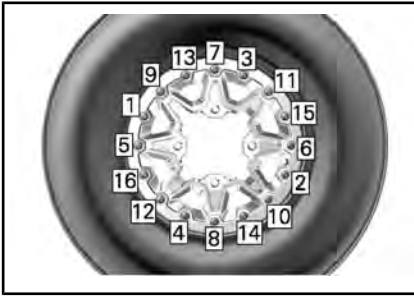
ТИПОВОЙ ВАРИАНТ - ПОРЯДОК ЗАТЯЖКИ ВИНТОВ
