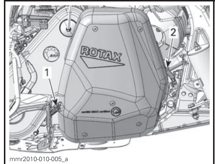
1. Пружины крепления выпускных труб к глушителю
