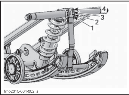
ТИПОВОЙ ВАРИАНТ 1. Положение 1 (заводская установка) 2. Положение 2 3. Положение 3 4. Положение 4
