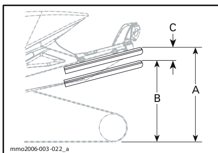
A. Максимально растянутая подвеска B. Подвеска под нагрузкой (вес водителя, пассажира и груза) C. Расстояние между величинами «А» и «В» ; обратитесь к таблице
