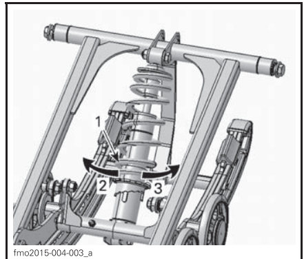
РЕГУЛЯТОР - ТИПОВОЙ ВАРИАНТ 1. Регулятор преднатяга пружины 2. Уменьшение преднатяга 3. Увеличение преднатяга
